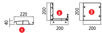
Lamelle coibentate e insonorizzate con poliuretano all'interno . Blades insulated and soundproofed with polyurethane inside
