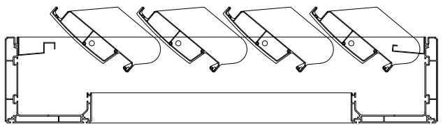
Rotazione lamelle a 140° . Blades rotation at 140°
