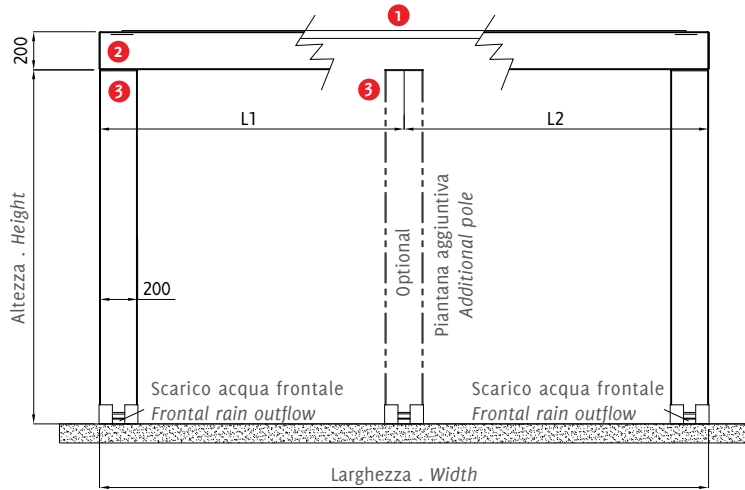
Lamelle coibentate e insonorizzate con poliuretano all'interno . Blades insulated and soundproofed with polyurethane inside
