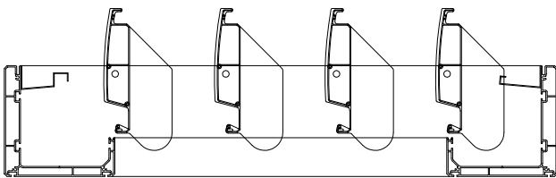
Rotazione lamelle a 90° . Blades rotation at 90°
