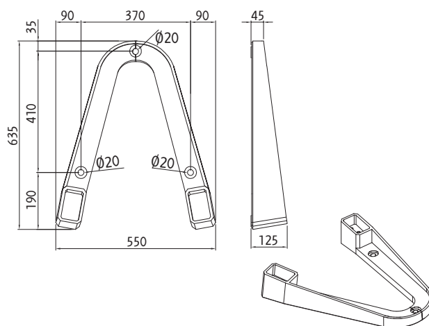
Piastra angolare a parete . Wall angular plate Regolazione da 0° a 50° . Adjustment from 0° to 50° 069-901
